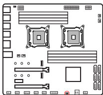
图2-1 清除CMOS跳线
