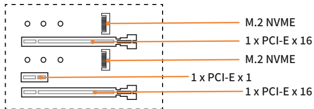
图2-4 PCI扩展插槽
